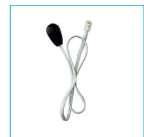
Deported IR
